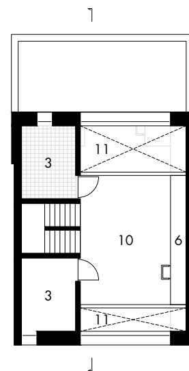
1E VERDIEPING
