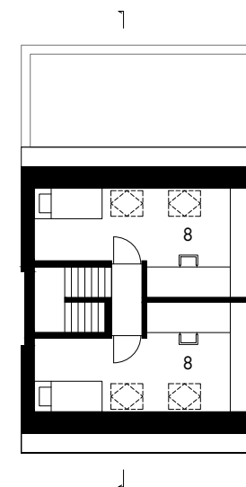
3E VERDIEPING
