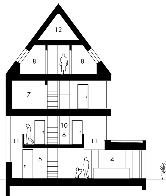
SNEDE
