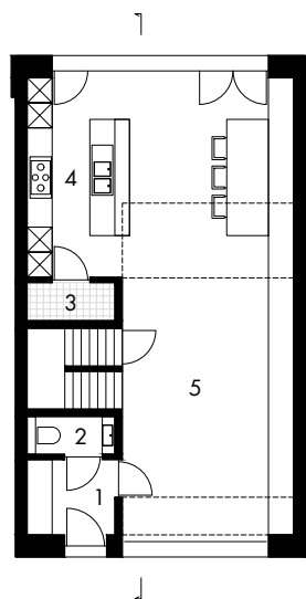
GELUJKVLOERS
