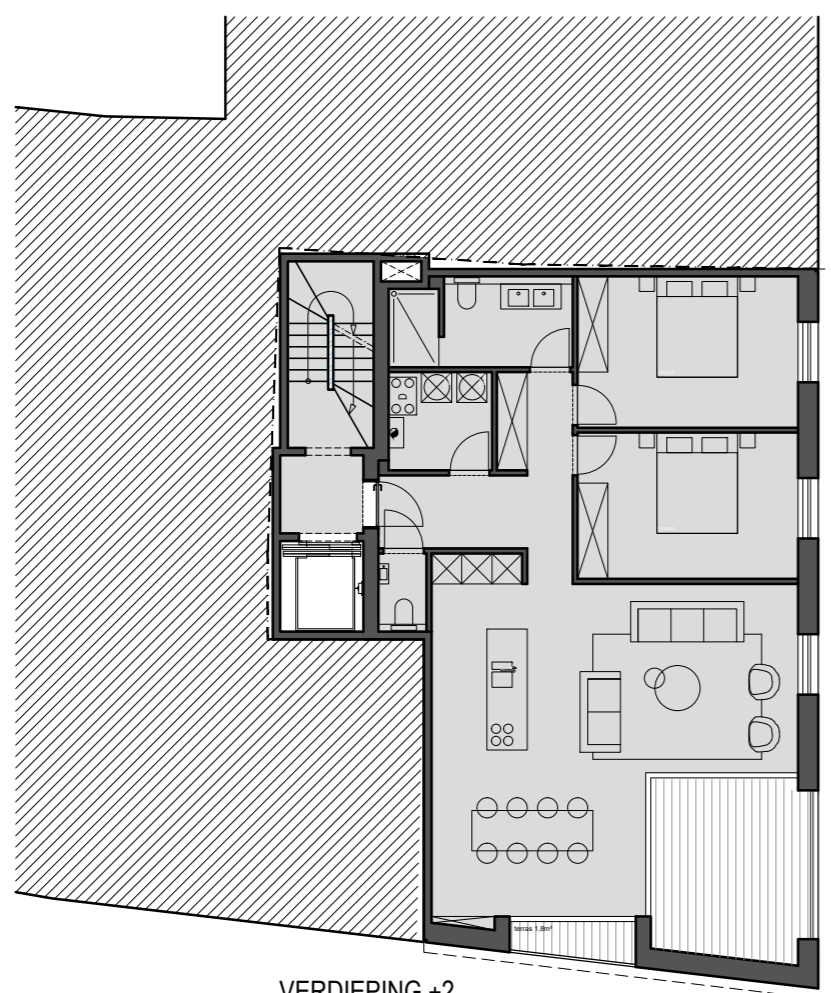
VERDIEPING +2
