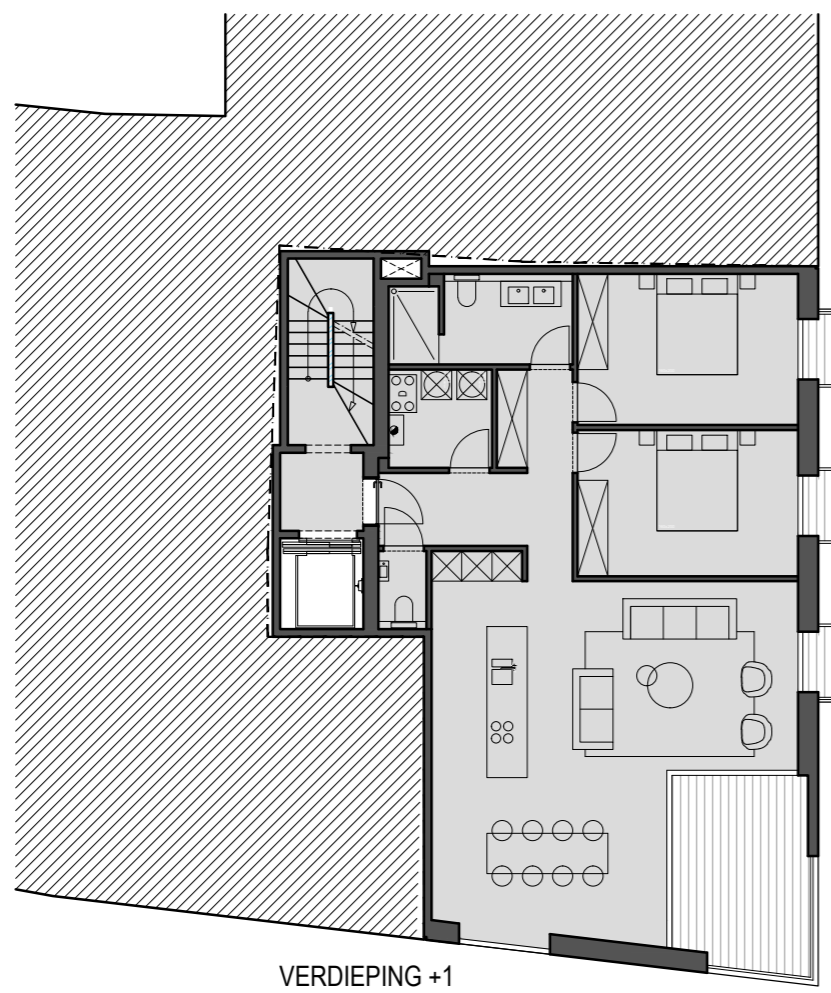
VERDIEPING +1
