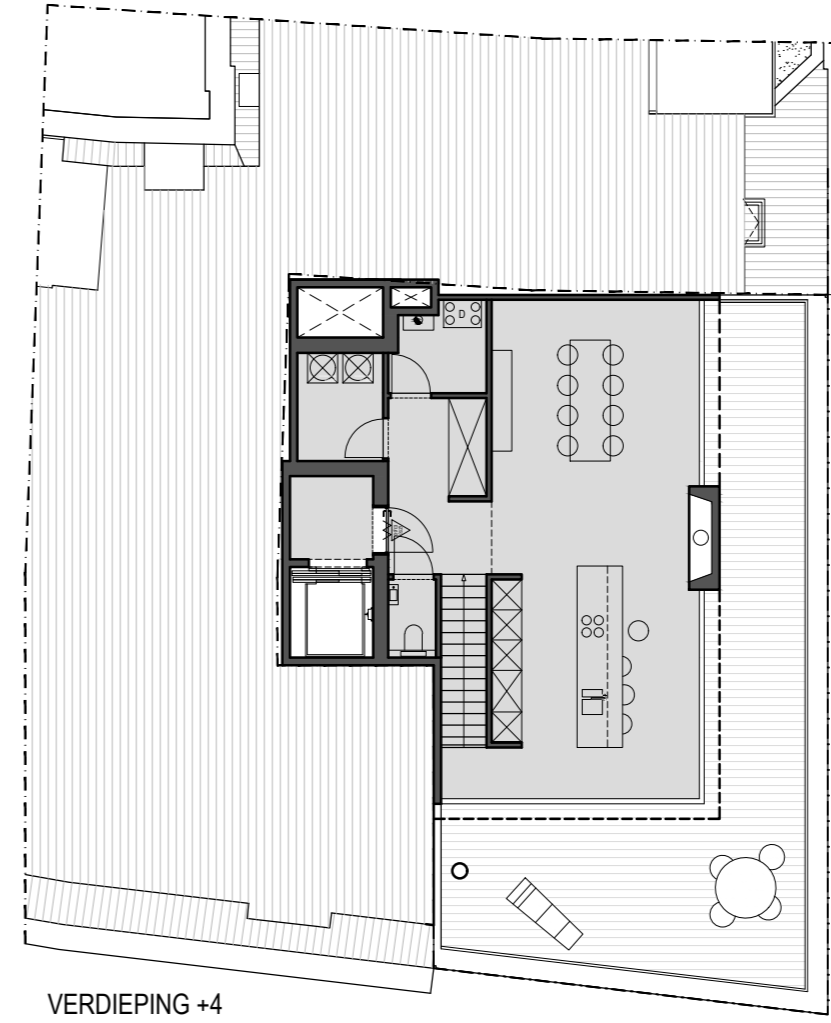
VERDIEPING +4
