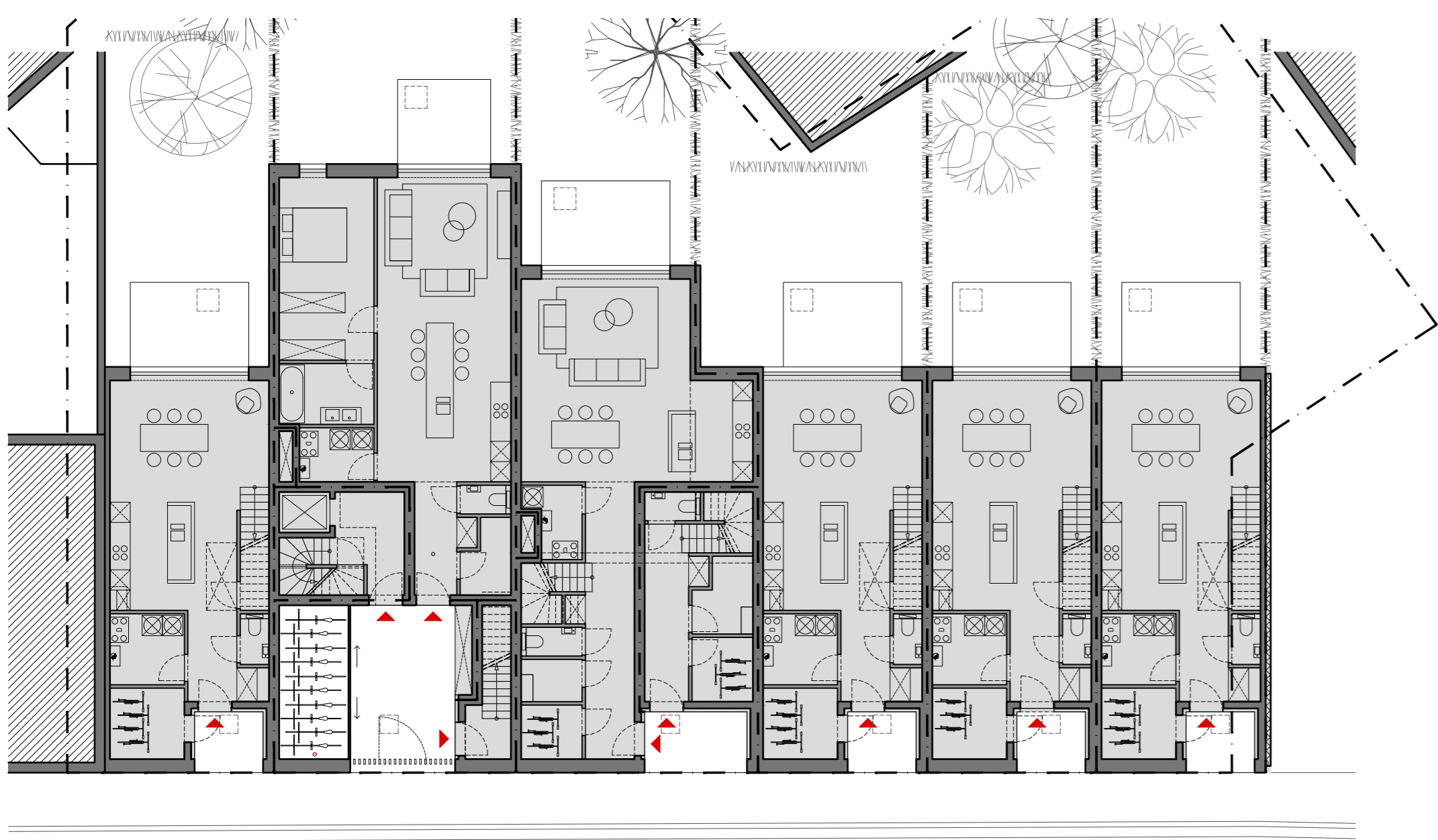
PLAN GELIJKVLOERS
