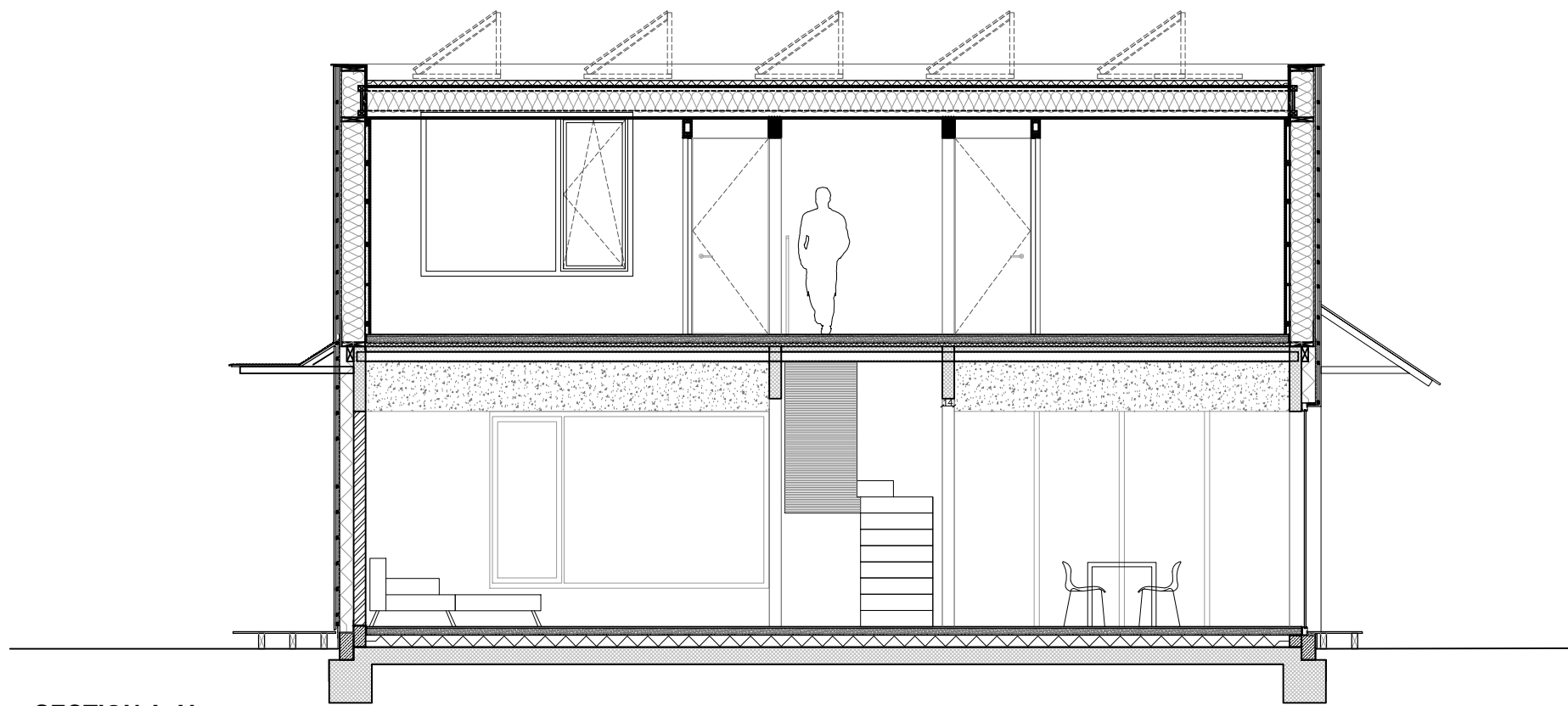
SECTION A-A'
