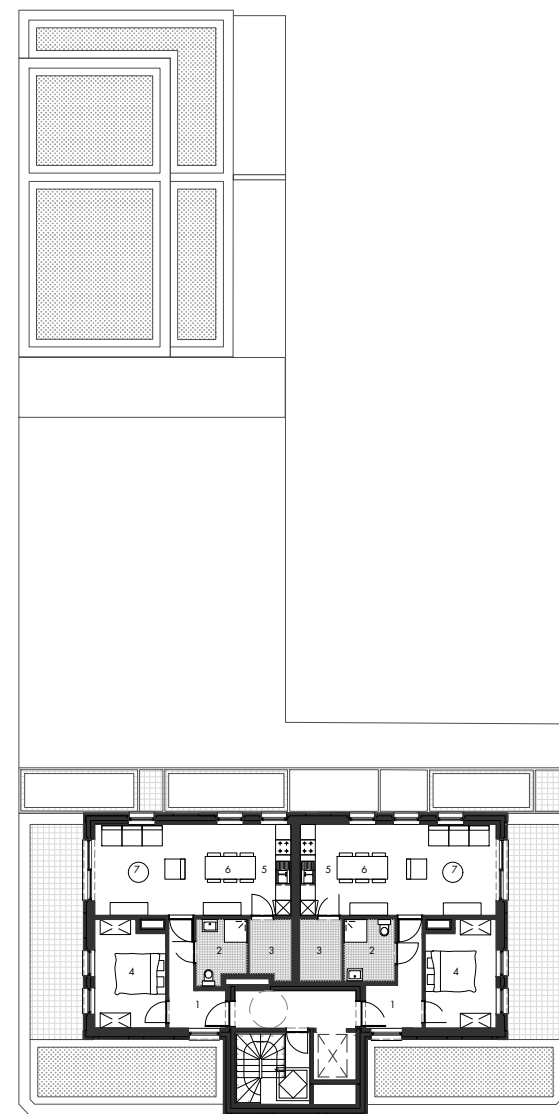
VIERDE VERDIEPING
