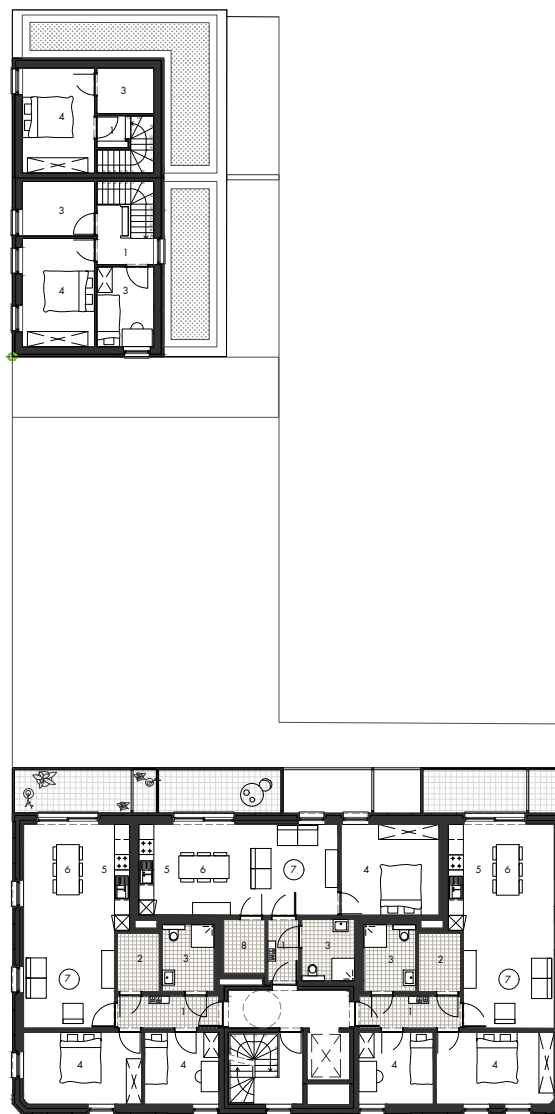
EERSTE VERDIEPING
