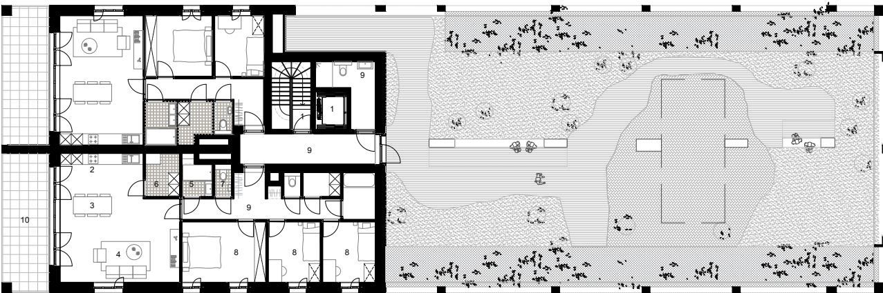
DERDE VERDIEPING
