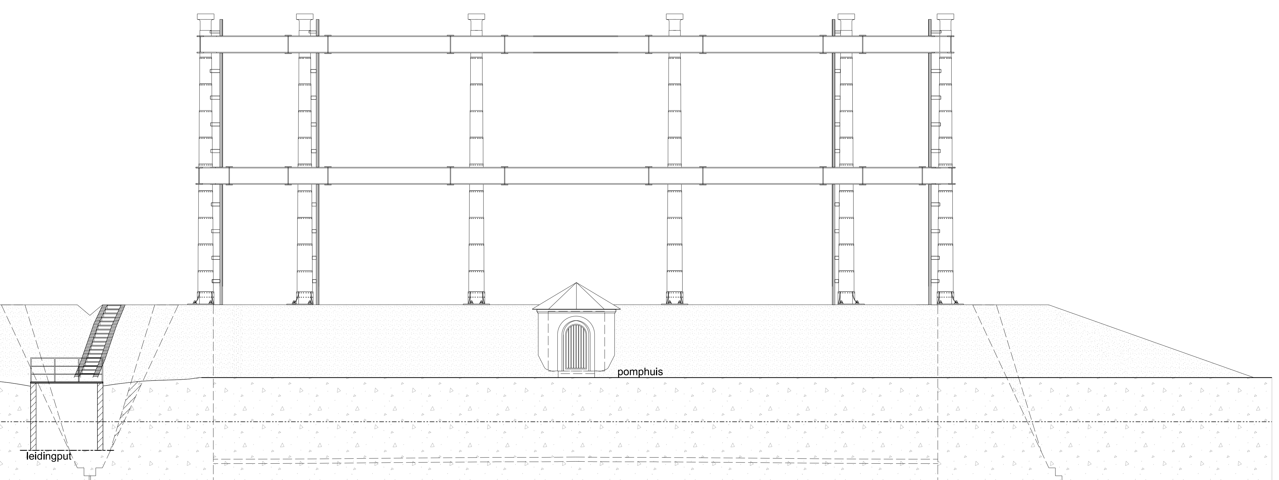
GASHOUDER 1 DOORSNEDE B - B
