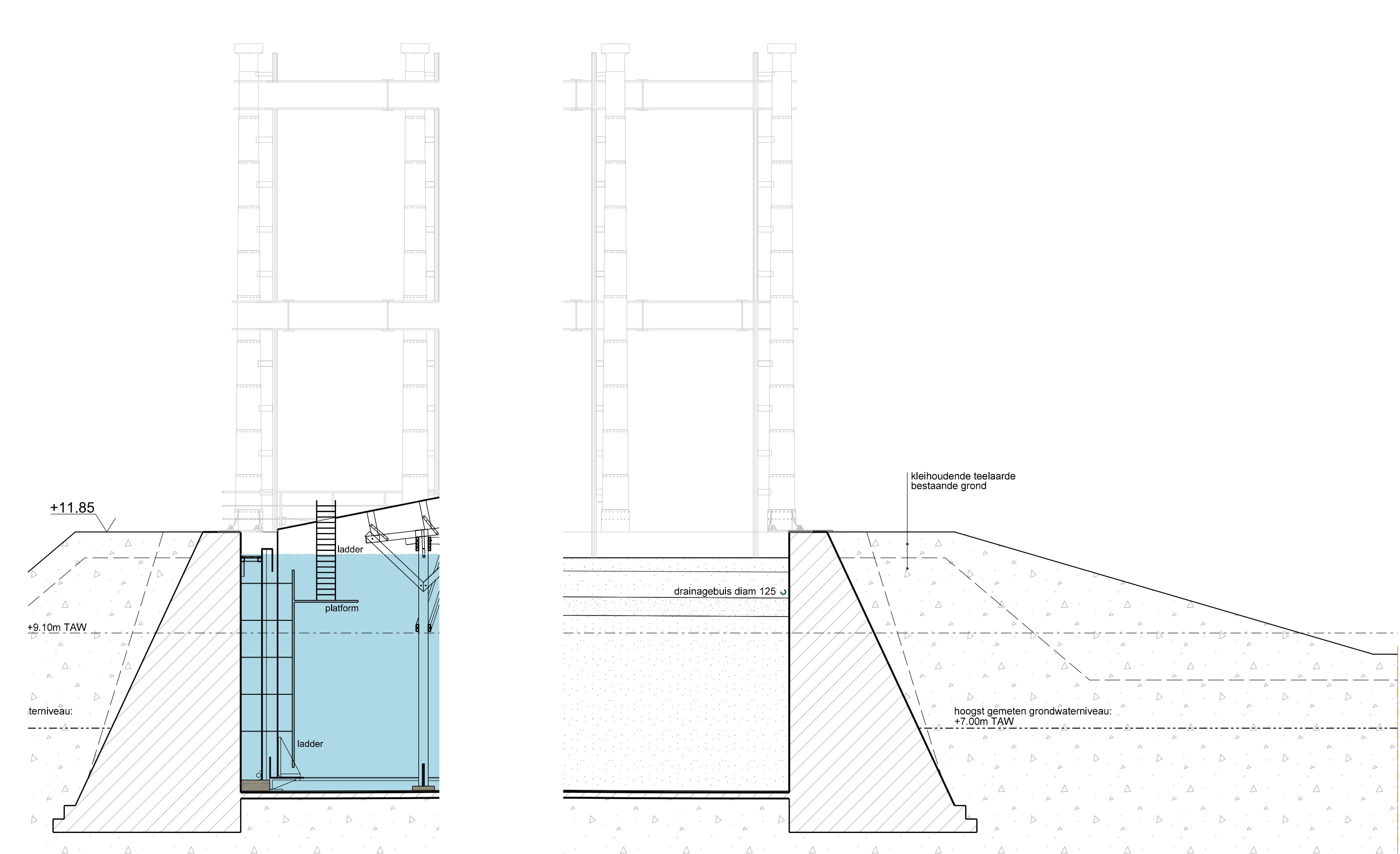
LADDER PRINCIPETEKENING
