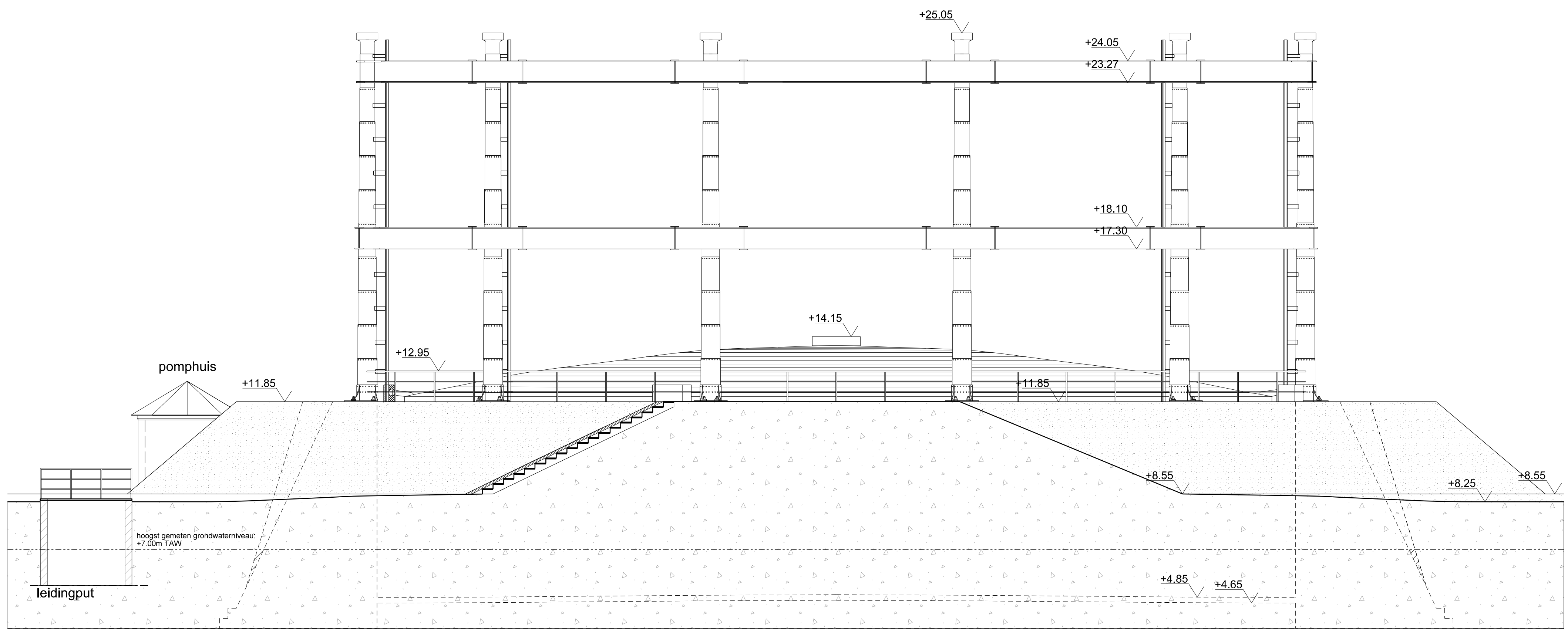
GASHOUDER 1 DOORSNEDE A - A
