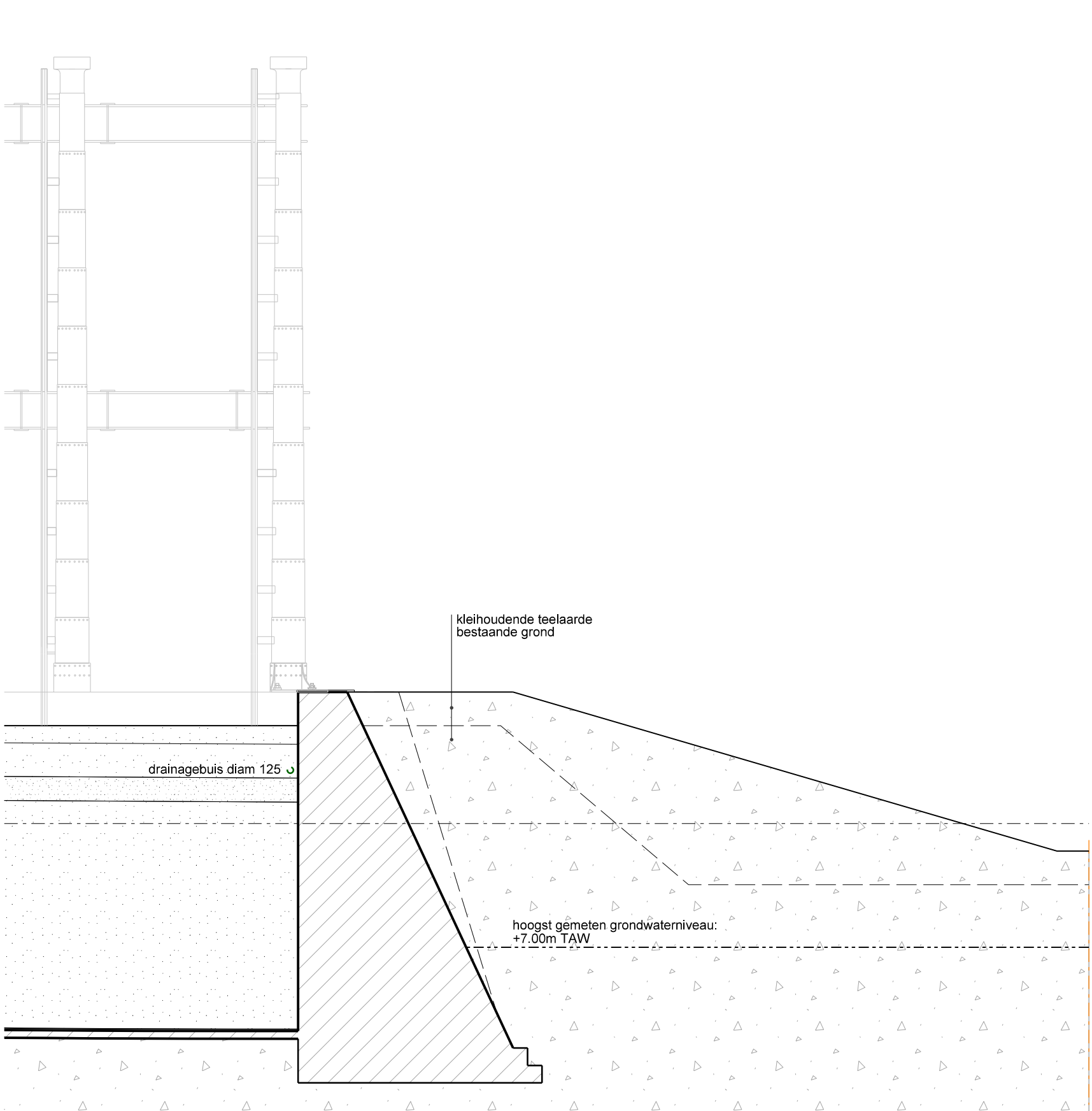
FLAUWE HELLING TALUD PRINCIPETEKENING
