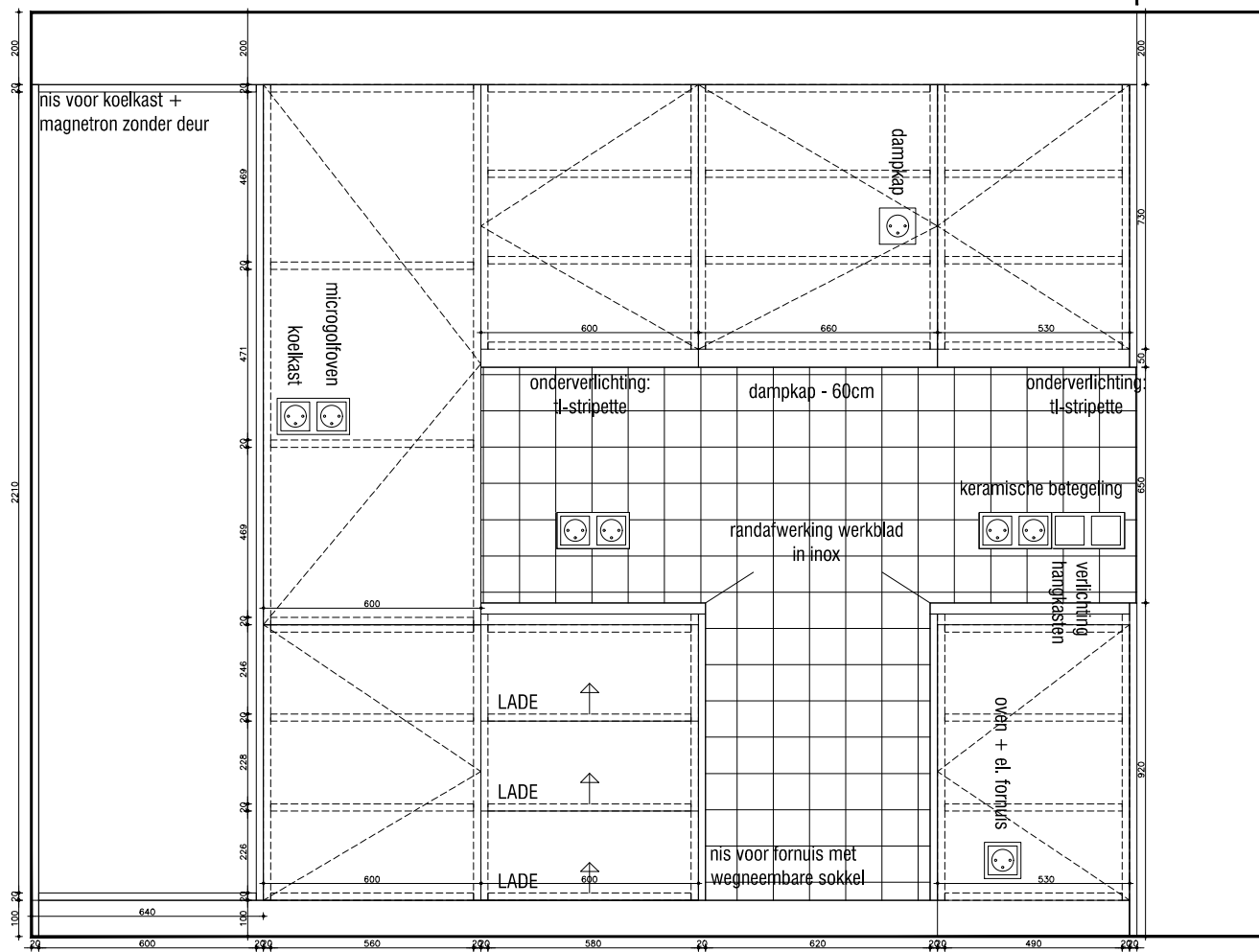
AANZICHT 1
