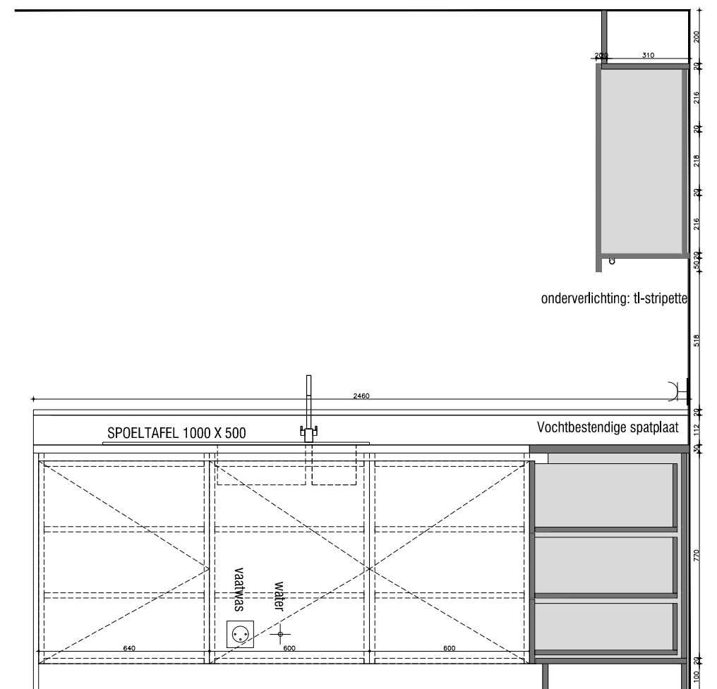
AANZICHT 2
