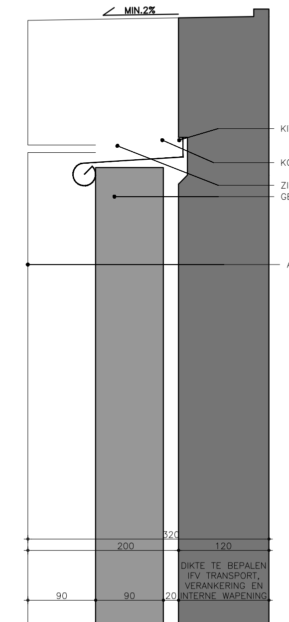
SNEDE 1
