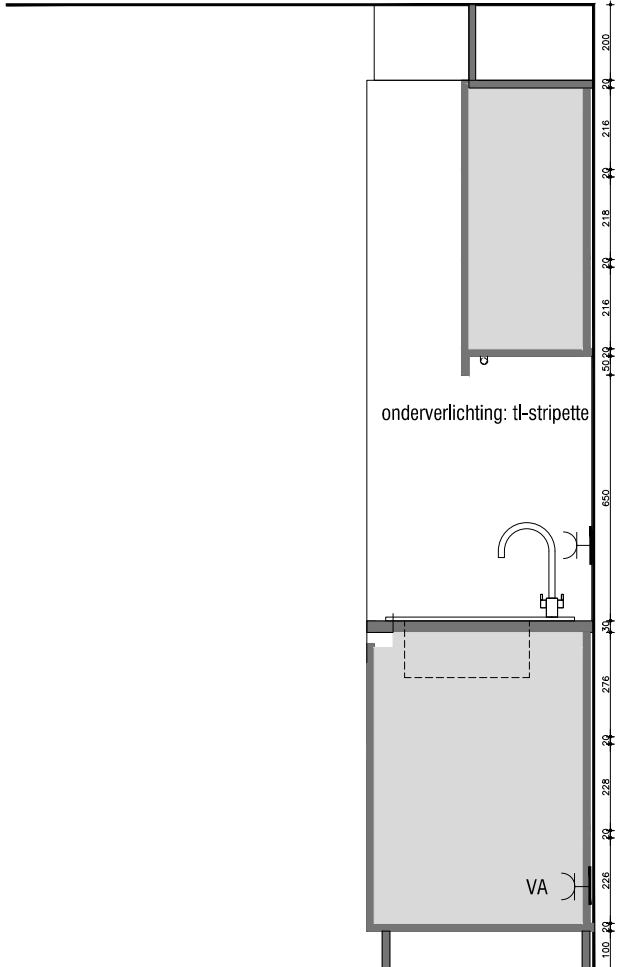
AANZICHT 2
