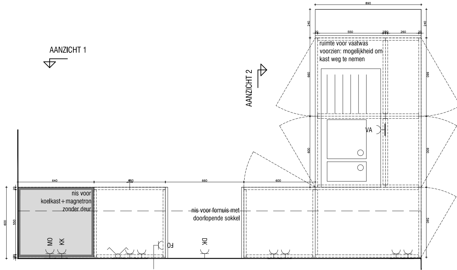
GRONDPLAN
