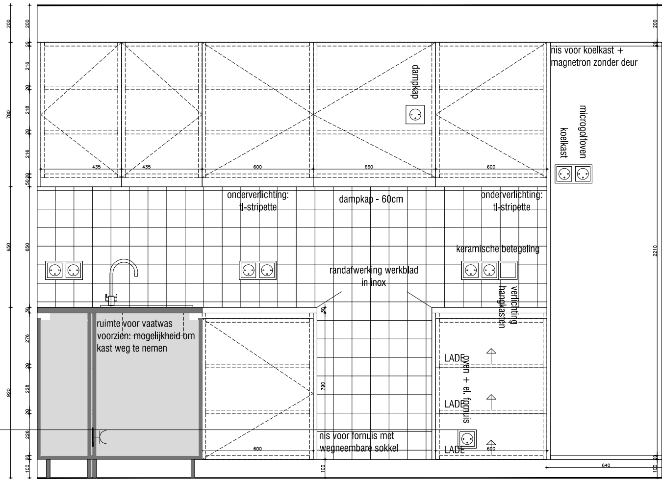
AANZICHT 1
