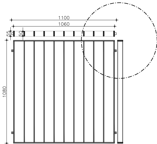
BALUSTRADE IN STALEN SPIJLTJES
