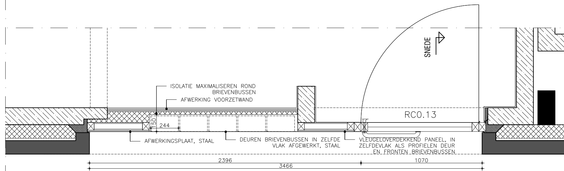
AANZICHT
