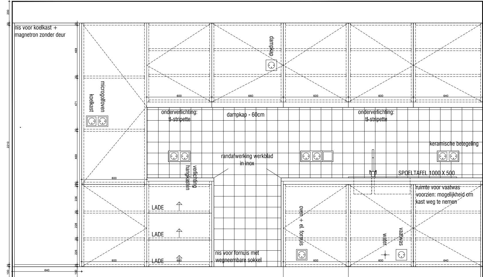
AANZICHT 1
