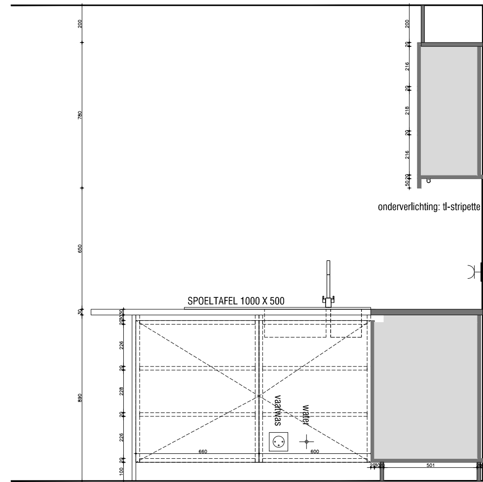
AANZICHT 2
