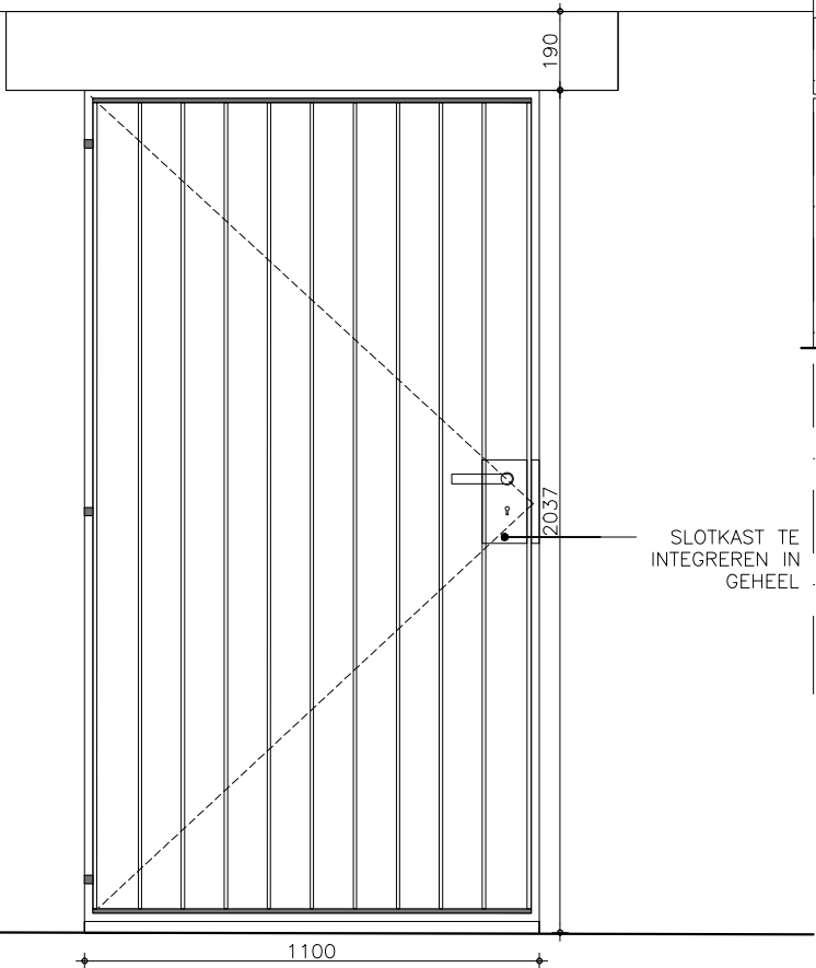
TUINPOORT T1 (TUINPOORT T2 IS SPIEGELBEELD VAN TUINPOORT T1)
