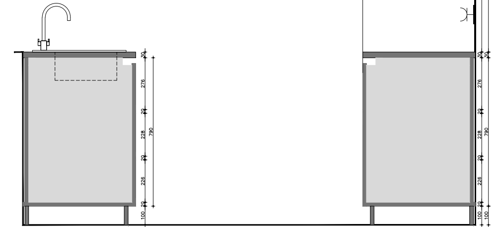
AANZICHT 3
