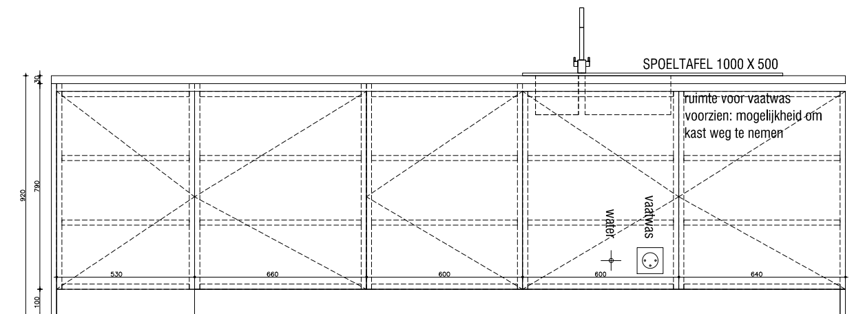
AANZICHT 2
