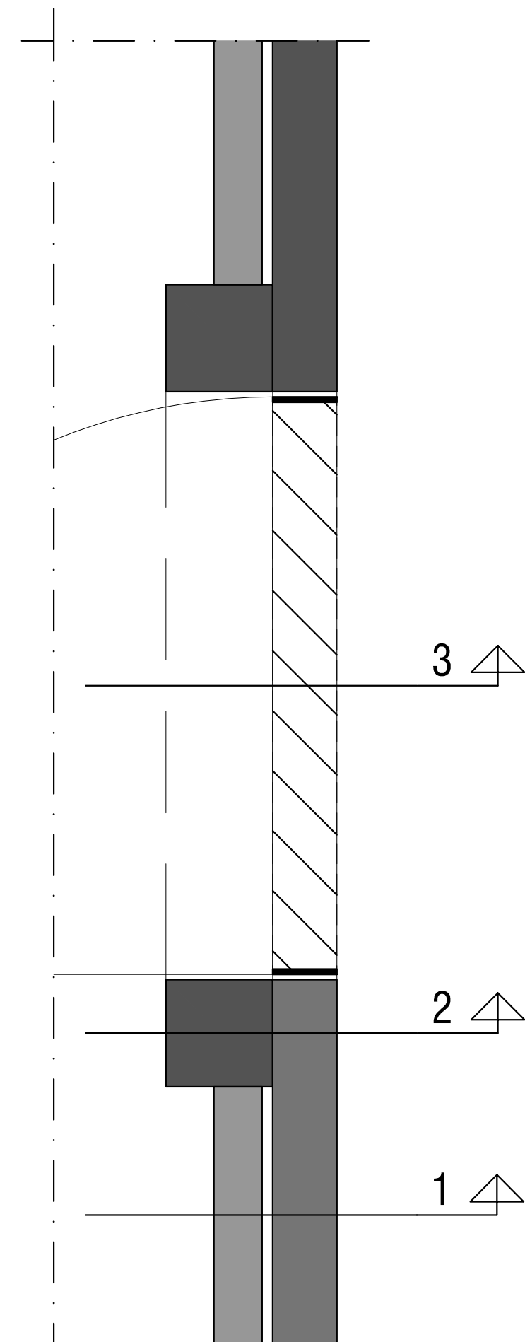
PLANSNEDE 1/10
