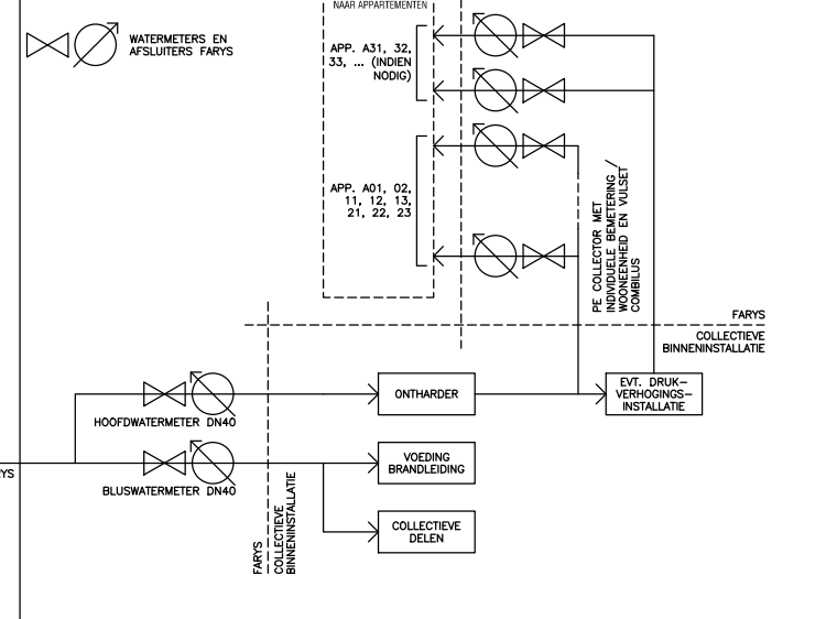
SCHEMATISCHE WEERGAVE AANSLUITINGEN WATER
