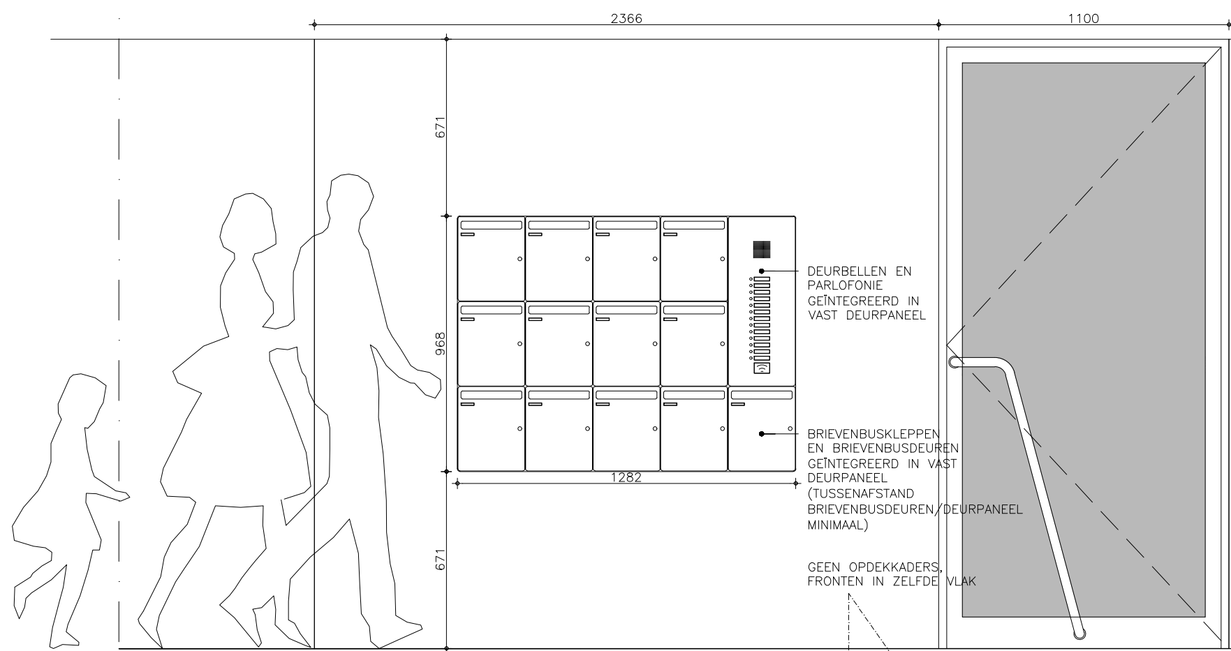
AANZICHT
