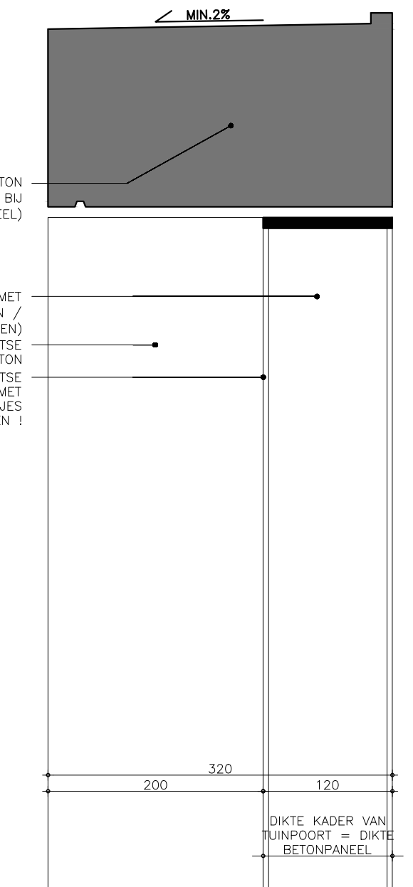
SNEDE 3
