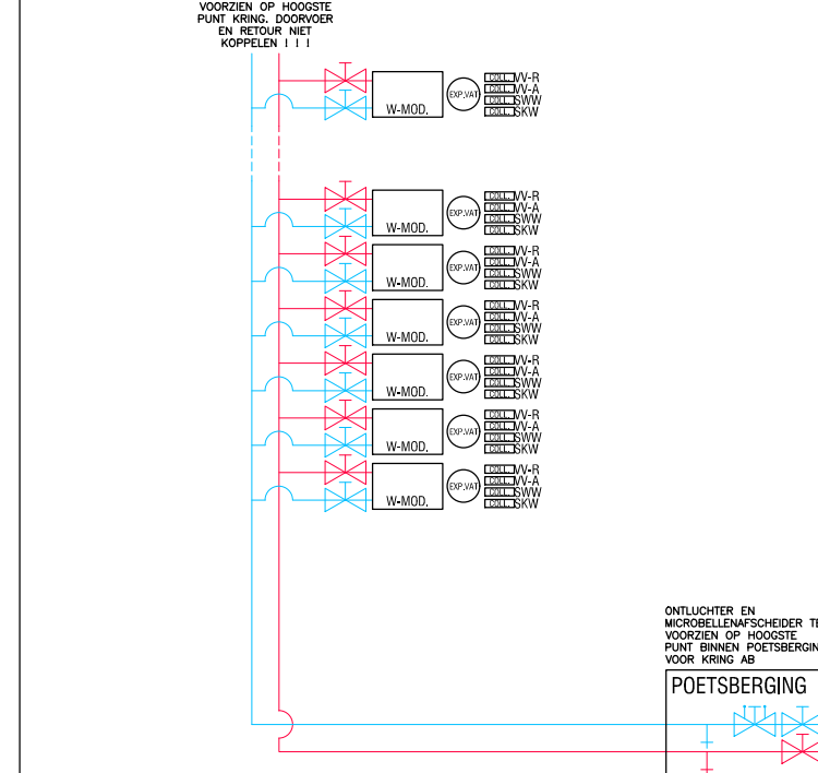
SCHEMATISCHE WEERGAVE COMBILUS
