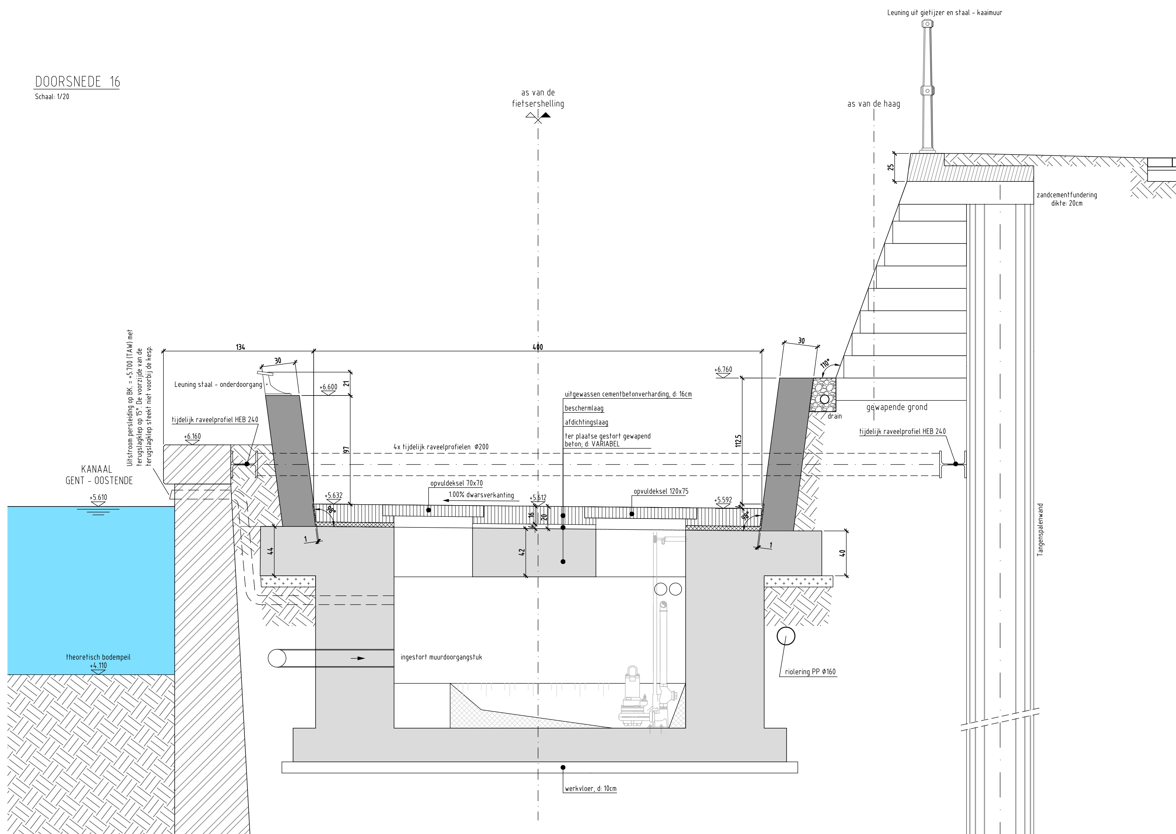
DOORSNEDE 19
