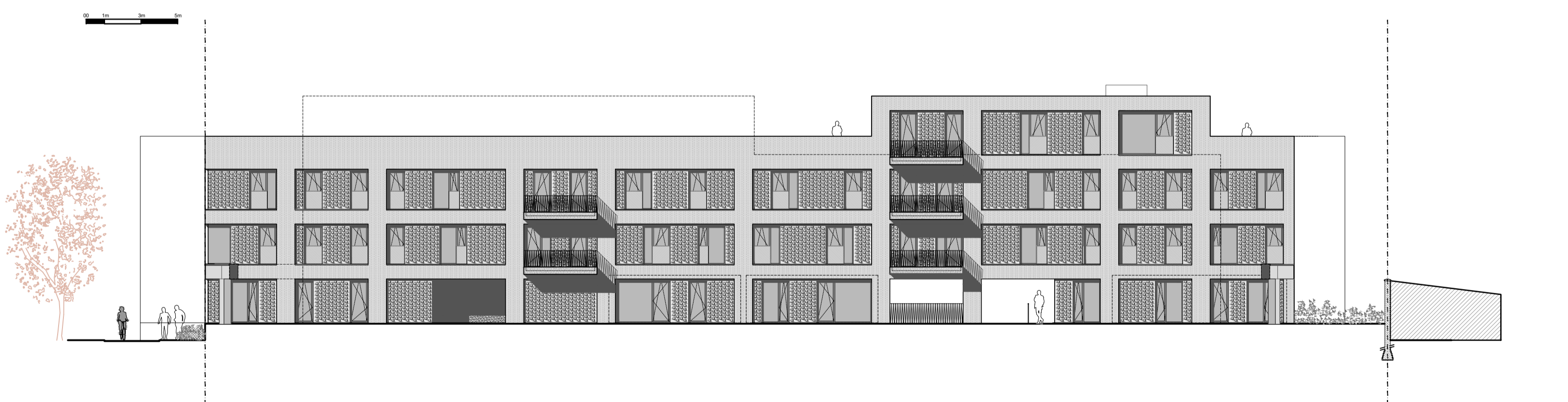
GEVEL BINNENGEBIED - GEBOUW A
