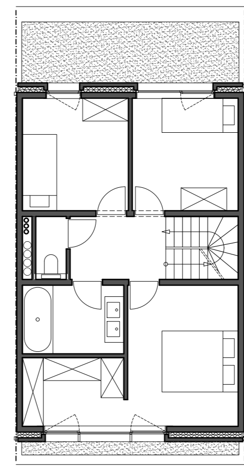
VERDIEPING 1
