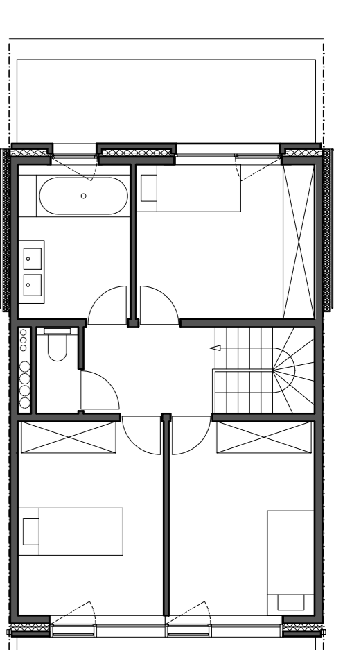
VERDIEPING 2
