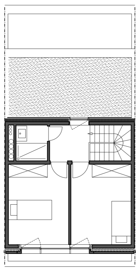
VERDIEPING 2
