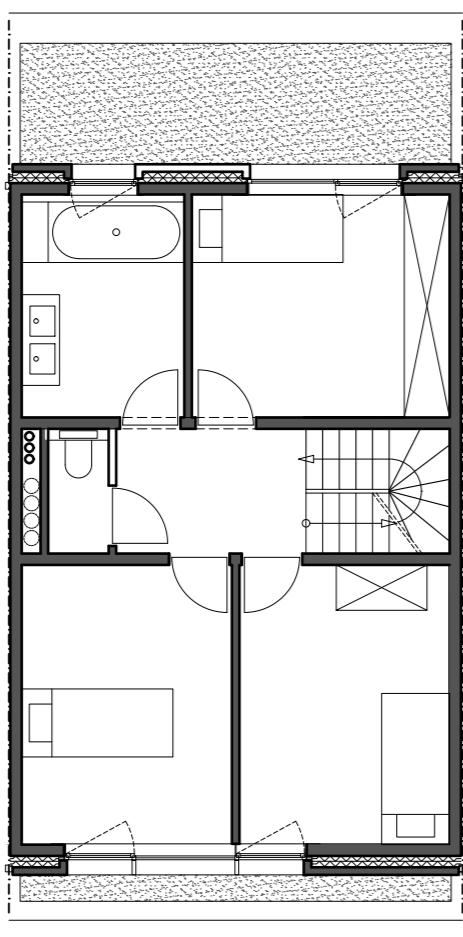
VERDIEPING 1
