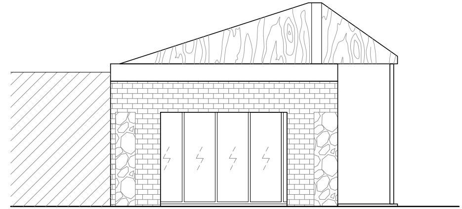
VOORGEVEL
