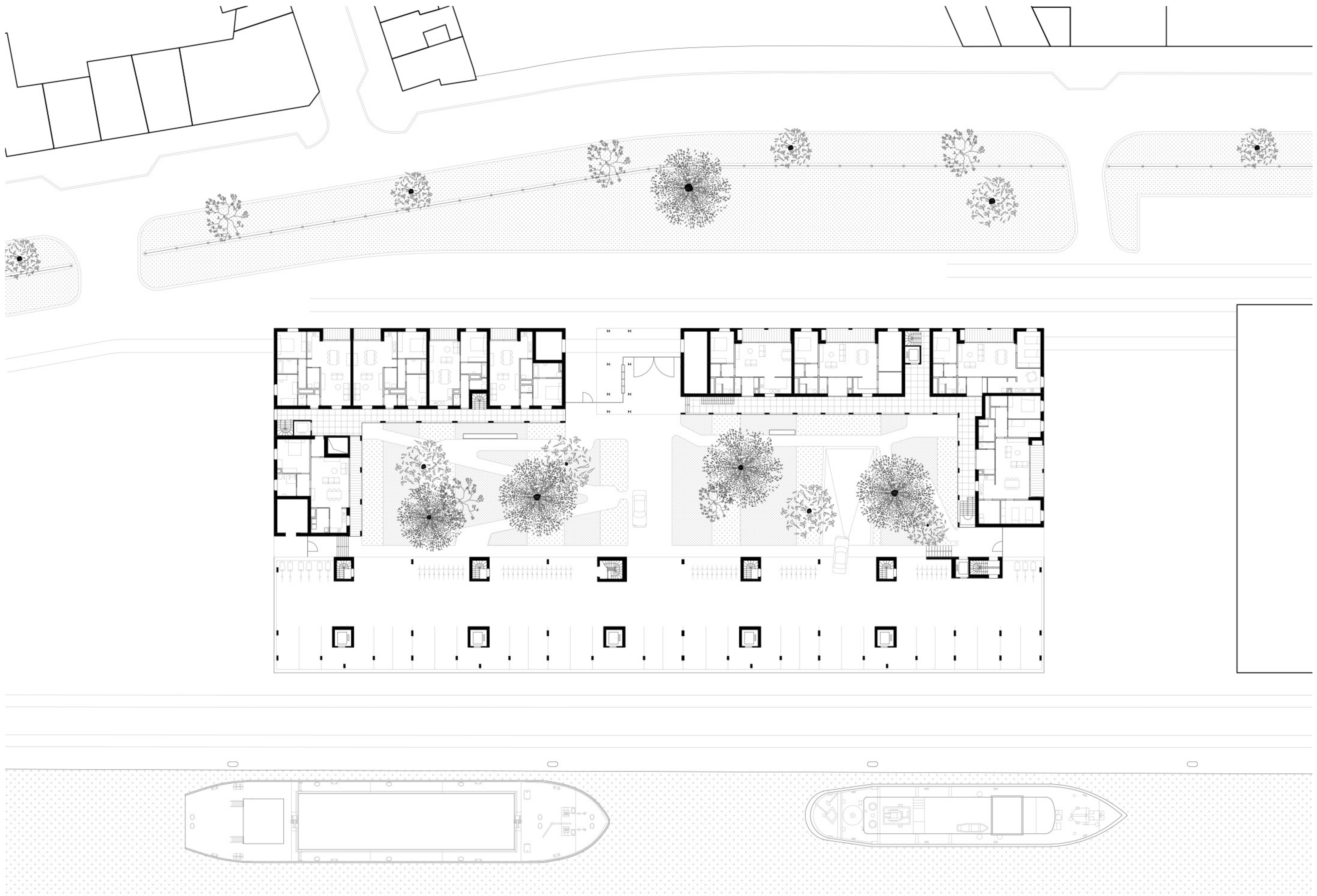
Plan gelijkvloers
