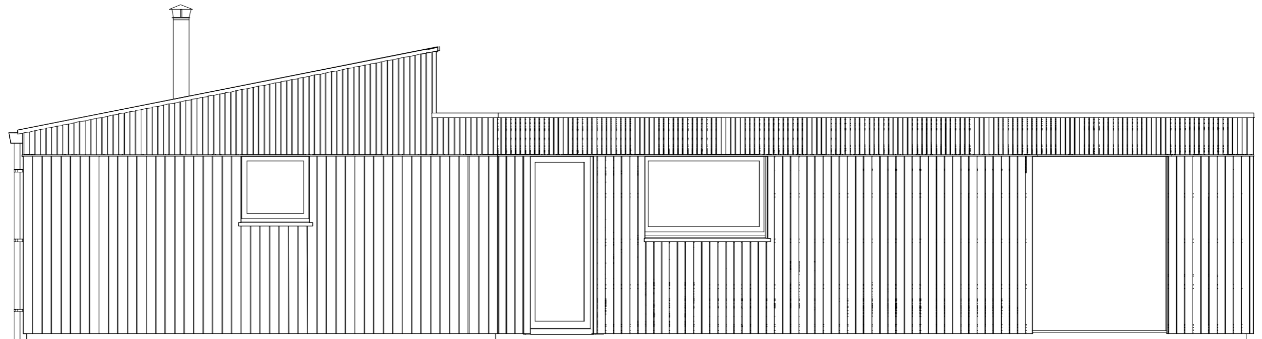
Oostgevel - nieuwe toestand schaal 1/50
