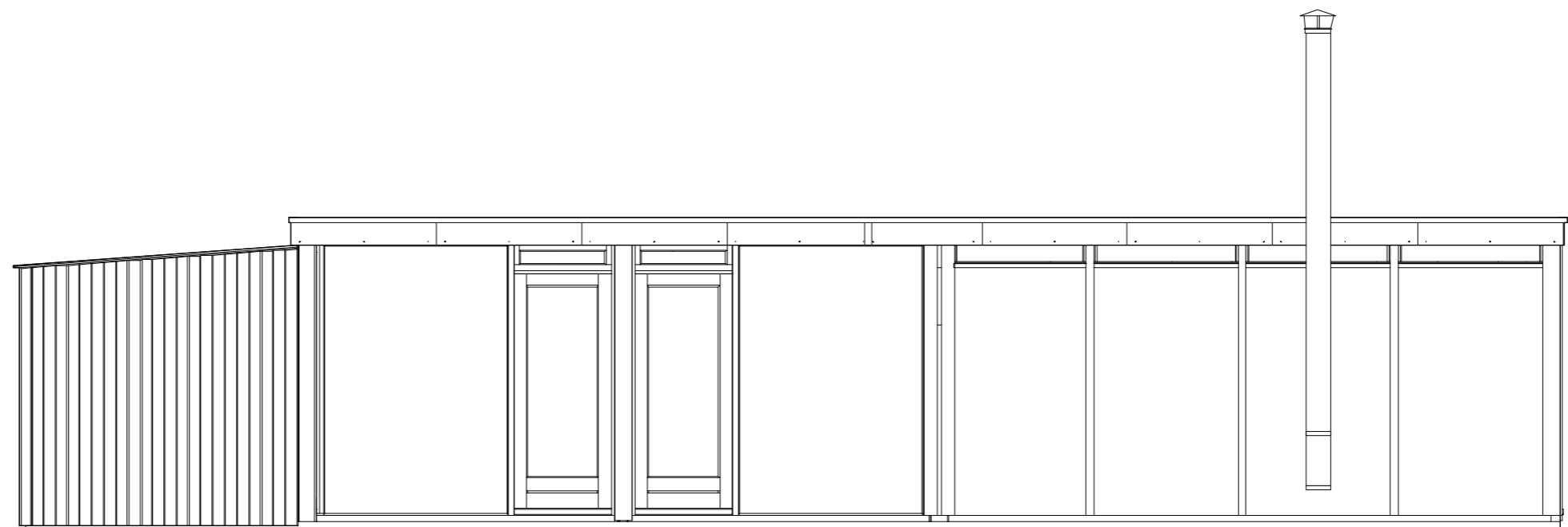
Westgevel - oude toestand schaal 1/50
