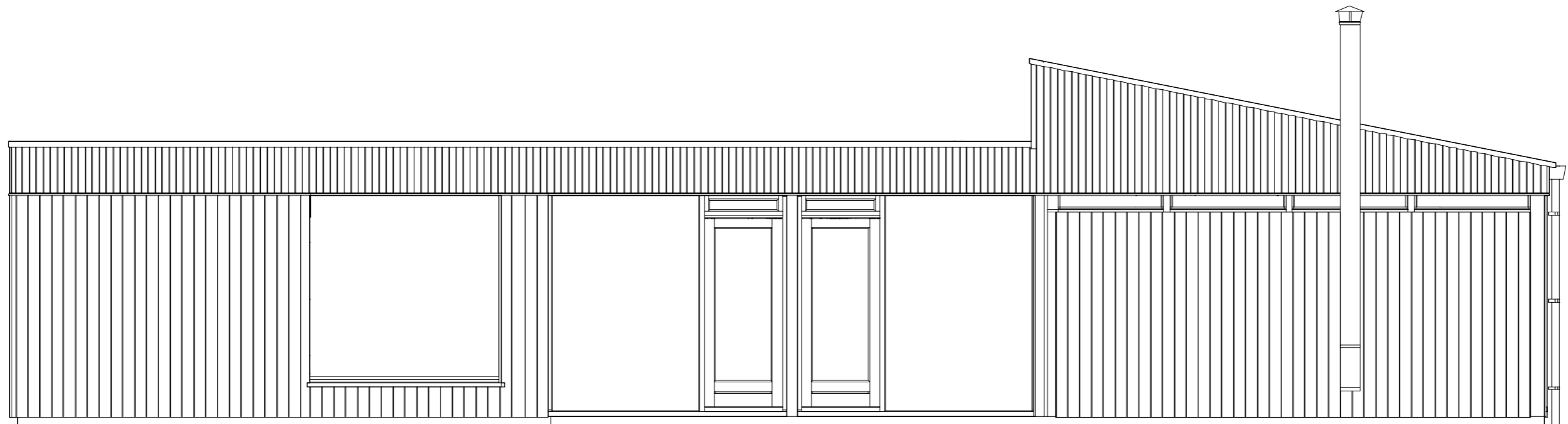
Westgevel - nieuwe toestand schaal 1/50
