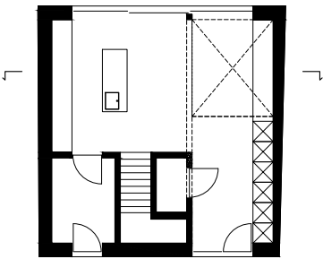
GELIJKVLOERS
