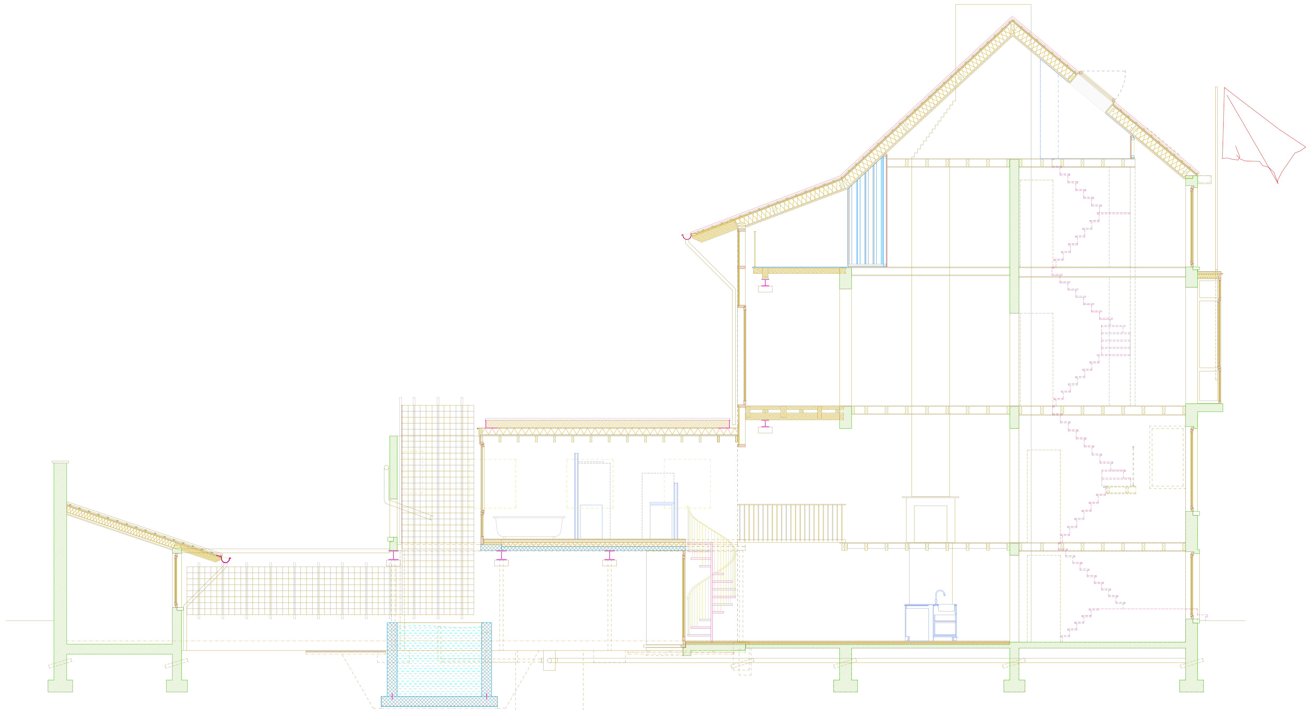
doorsnede BB', nieuwe situatie
