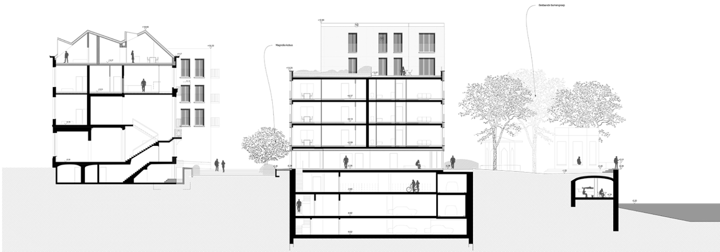
SNEDE I - DWARSE SNEDE GEBOUW C / D / PAVILJOEN
