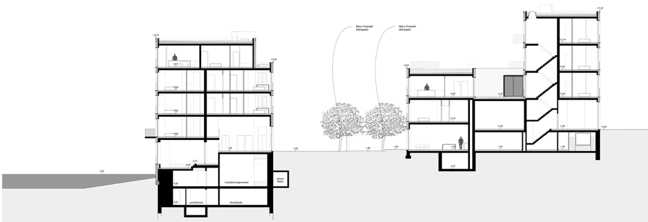
SNEDE M - DWARSE SNEDE GEBOUW E / F
