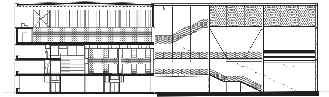
snede A-A'
